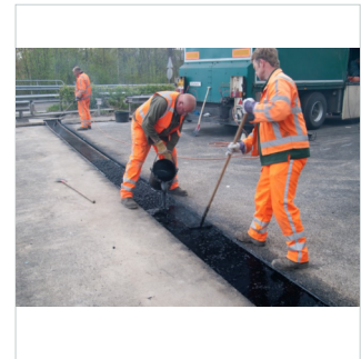
aanbrengen voegmassa
