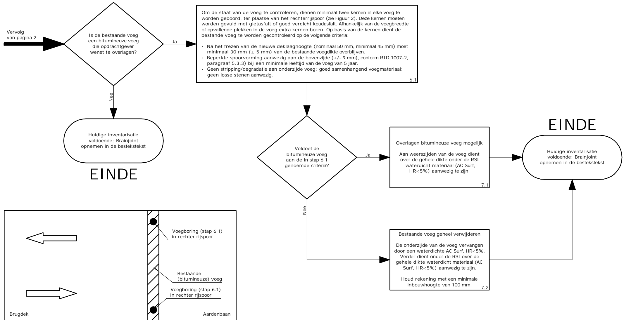
Figuur 2; prinsesochets voegboringen (stap 6.1)
