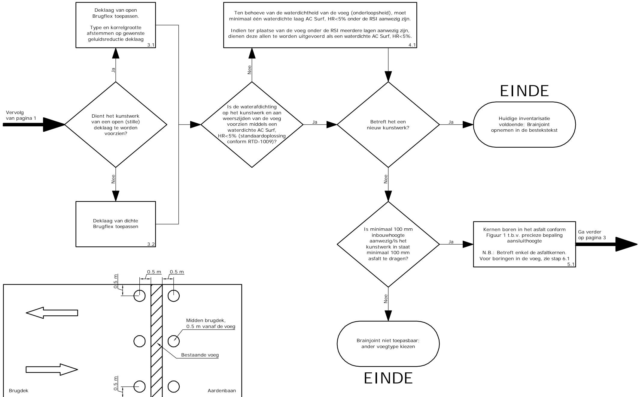
Figuur 1; prinseschems asfaltboringen (stap 5.1)
